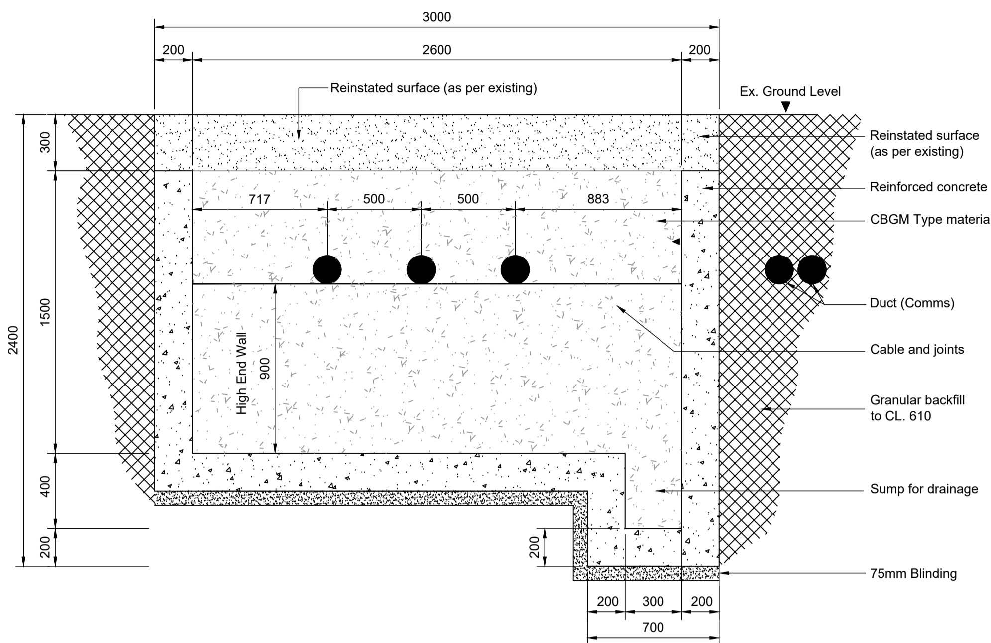
Section A-A 1:20
